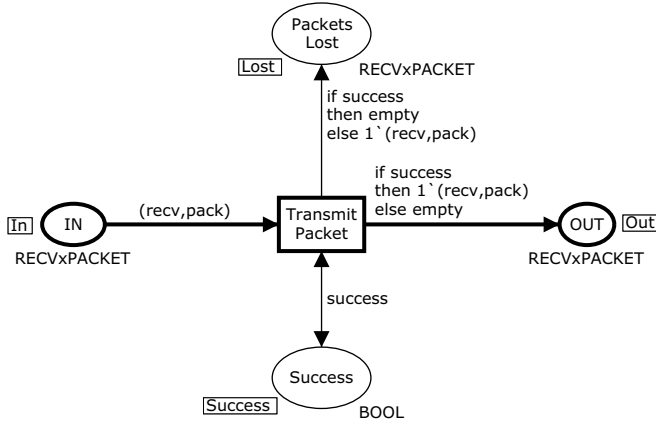
Fig. 6.5 Transmit module
