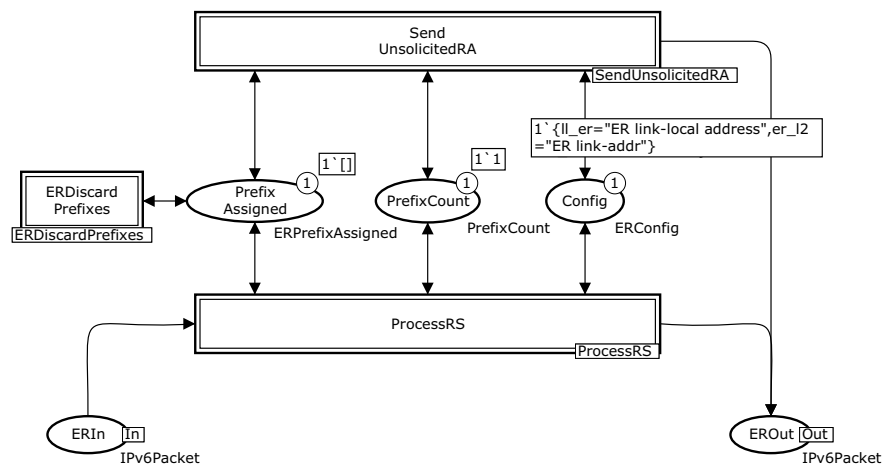
Fig. 14.6 EdgeRouter module
