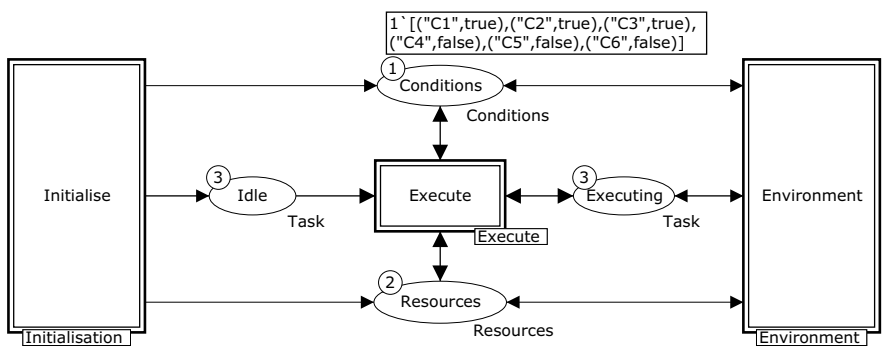
Fig. 14.33 CoastServer module
